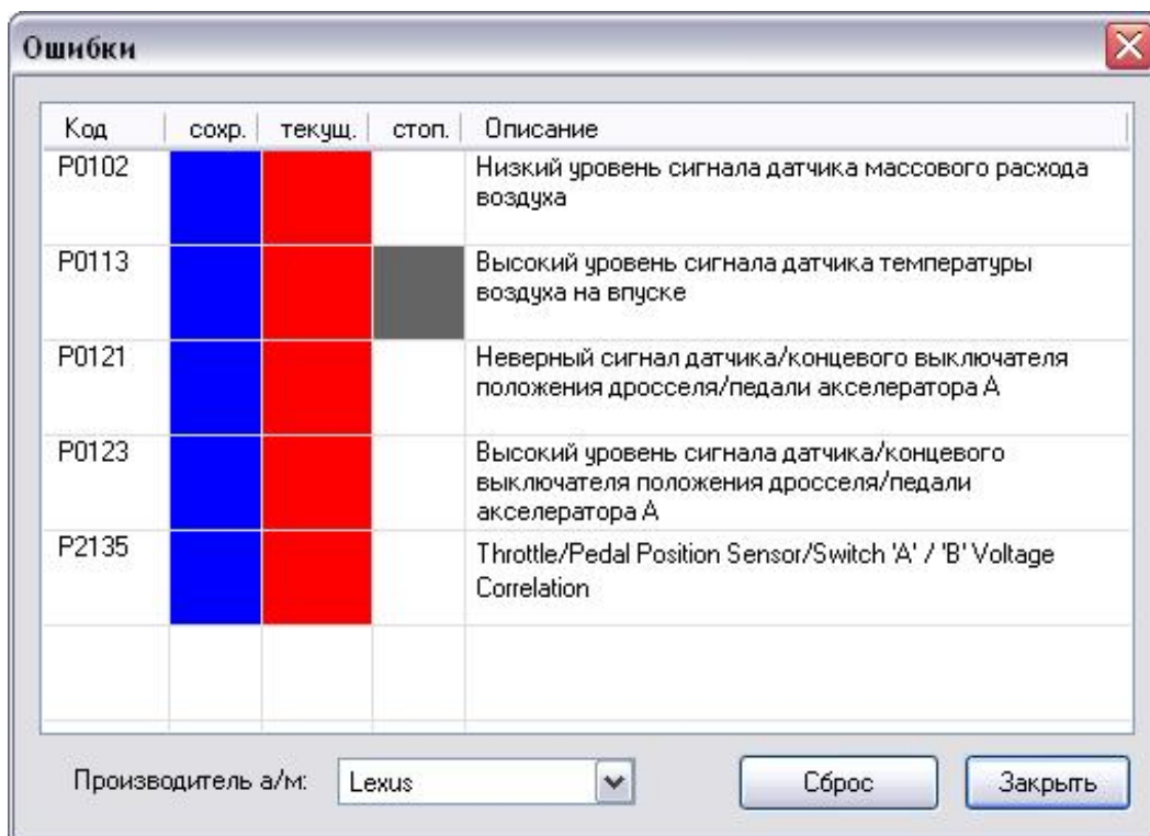
Рис. 6. Окно "Ошибки".
